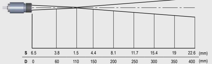
CF optics, D:S = 75:1
