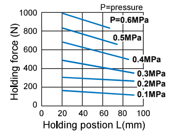
MCHG2-125
