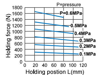
MCHG2-125
