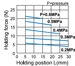
MCHG2-20
