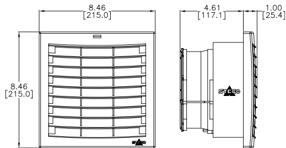
6.93 x 6.93 in Cutout Size FPO Fan
