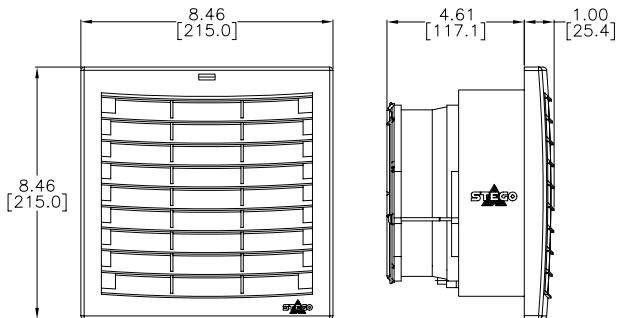
6.93 x 6.93 in Cutout Size FPI Fan
