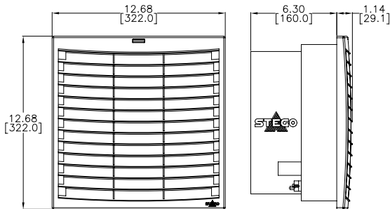
11.46 x 11.46 in Cutout Size FPI Fan
