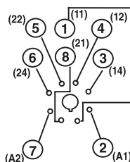
750-2C-SKT
