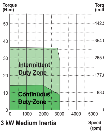
Servo Drive SVA-2300 <-->
