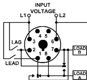
ARX-2C-120A
