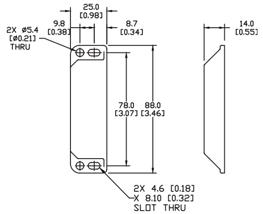
ACTUATOR
