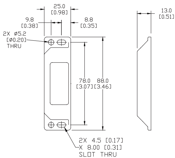
ACTUATOR
