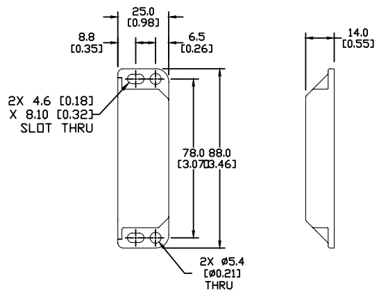
ACTUATOR
