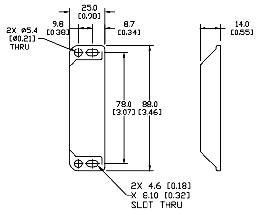
ACTUATOR
