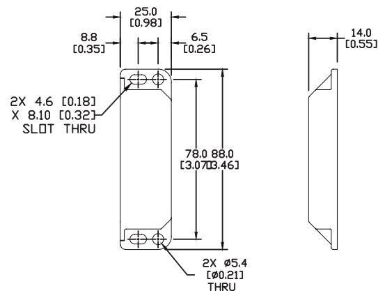
ACTUATOR
