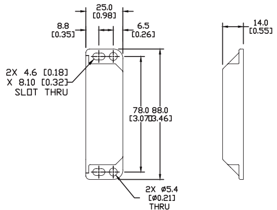
ACTUATOR
