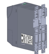
Figure A2: (a) Detach the fixation snaps by screws (a) Destacar las trabas de fijación por tornillos (a) Destacar as travas de fixação por parafusos
