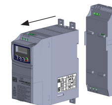
Figure A2: (b) Fit the filter set on the CFW300 base (b) Encaje el conjunto filtro en la base del CFW300 (b) Encaixe o conjunto filtro na base do CFW300
