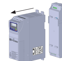
(b) Encaixe o conjunto filtro na base do CFW300
