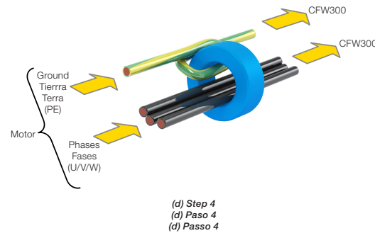
Figure A6: (a) to (d) Common mode choke installation on the motor cables Figura A6: (a) a (d) Instalación del choke de modo común en los cables del motor Figura A6: (a) a (d) Instalação do choke de modo comum nos cabos do motor
