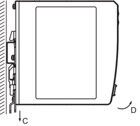
Figure 2 : démontage
