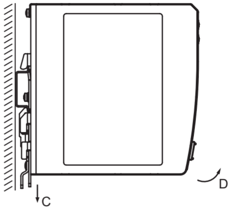
Abbildung 2: Demontage
