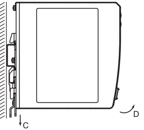
Рис 2: демонтаж
