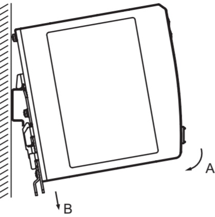
Рис 1: монтаж
