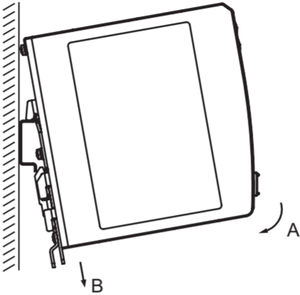
Рис 1: монтаж
