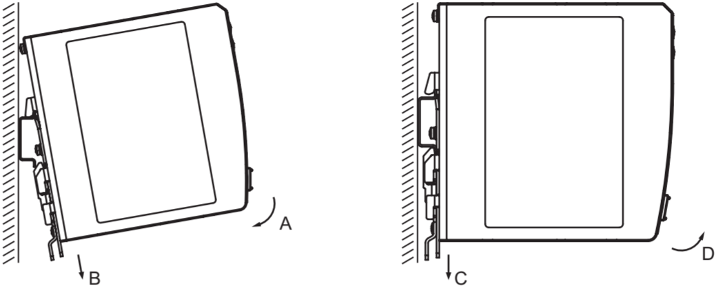
Abbildung 1: Montage
