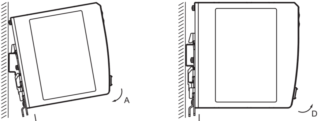
Abbildung 1: Montage
