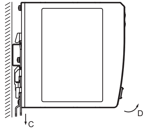
Abbildung 2: Demontage
