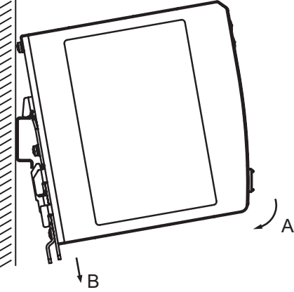
Рис 1: монтаж
