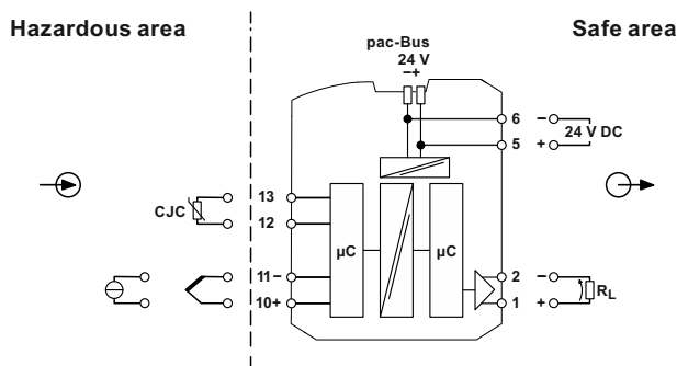
Prinzipialschaltbild 9282/12-51-16
