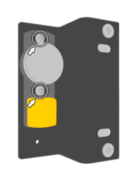
Abb.5: Ankerplatte an Montageplatte anbringen und Schrauben M6 x 8 mm Torx festziehen.
