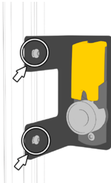
Abb.8: Montageplatte mit Prozesszuhalterung am Profil anbringen und und Schrauben M8 x 12 mm Torx festziehen.
