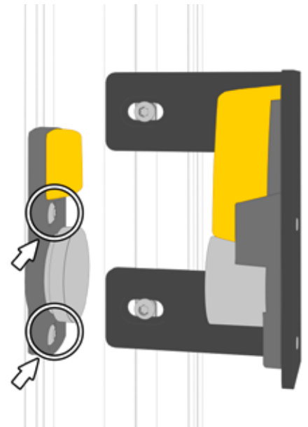
Abb.9: Ankerplatte am Profil der Schiebetüre anbringen, zur Prozesszuhalterung ausrichten und zur Prozesszuhalterung ausrichten. Schrauben M6 x 16 mm Torx festziehen.
