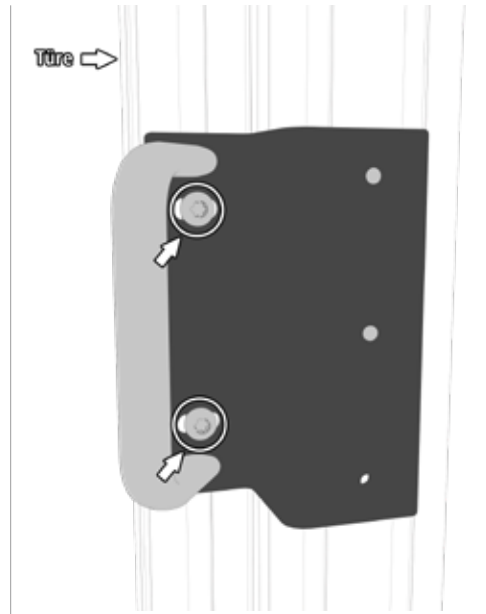
Abb.6: Montageplatte mit Ankerplatte am Profil anbringen und zur Prozesszuhalterung ausrichten. Schrauben M8 x 12 mm Torx festziehen.
