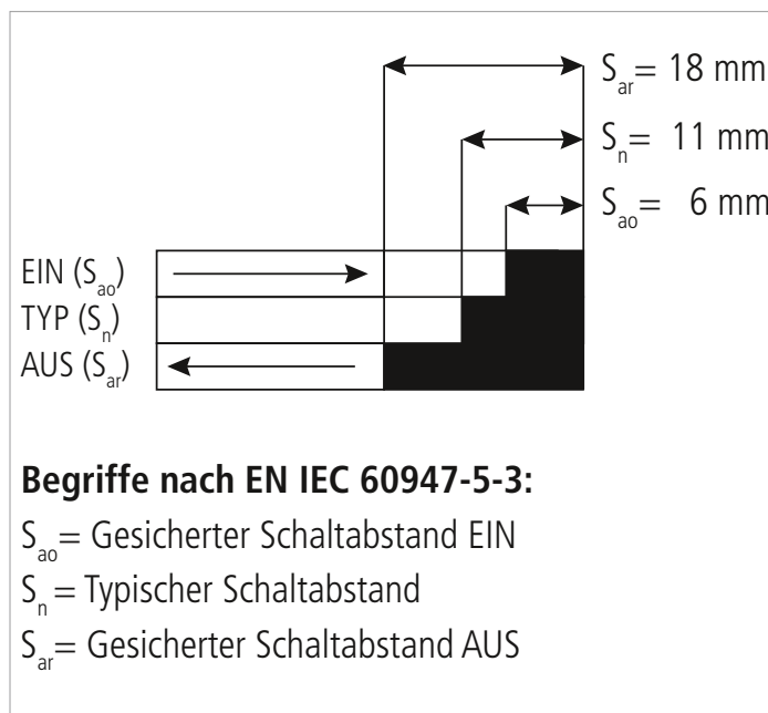
Abb.12: Schaltabstand
