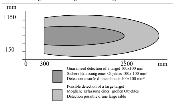
Wiring/Anschlüsse/Raccor dement électrique Detection range / Erfassungsbereich/ Plage de détection mm
