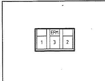
Links: EFM/ELM Rechts: Querschnitt EFM/ELM 1 Flanschbefestigungsschrauben 2 Montageflansch für drei Kontaktelemente
