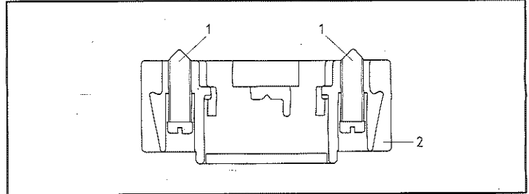
À gauche: EFM/ELM À droite: Coupe transversal EFM/ELM 1 Vis de fixation des brides 2 Brides de montage pour trois éléments de contact
