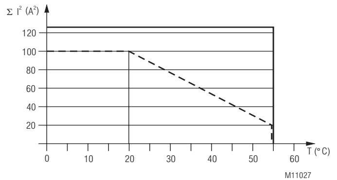
Courbe limite de courant totalisateur AC 230 V
