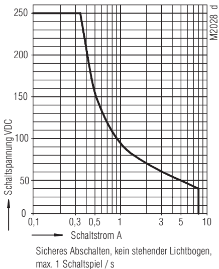
Lichtbogengrenzkurve
