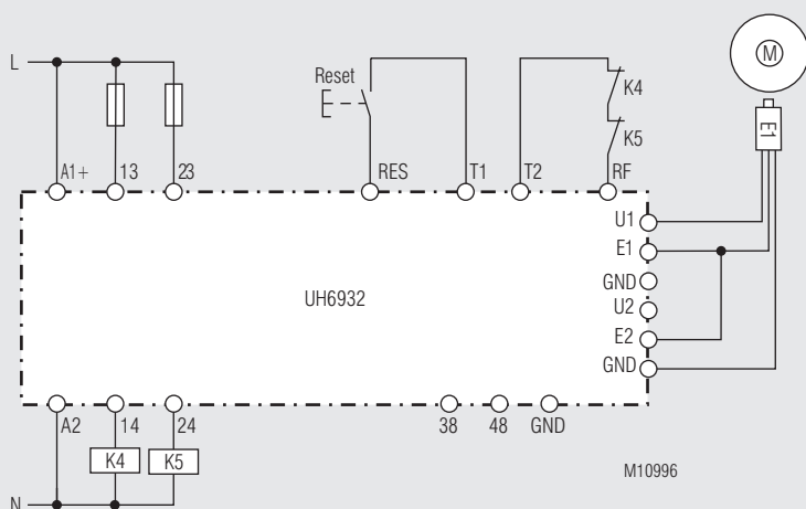
Raccordement avec un initiateur, convient jusqu'à SIL2, Performance Level c, Cat. 2 (Une condition primordiale pour le maintien de la catégorie 2 est le contrôle à intervalles réguliers de la fonction de sécurité)
