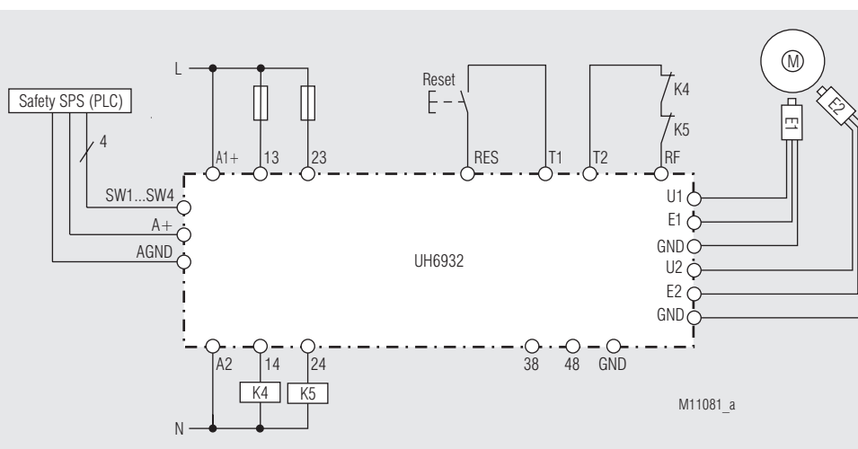
Raccordement standard avec UH6932/_ _1, convient jusqu'à SIL3, Performance Level e, Cat. 4
