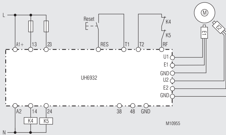
Raccordement standard, convient jusqu'à SIL3, Performance Level e, Cat. 4
