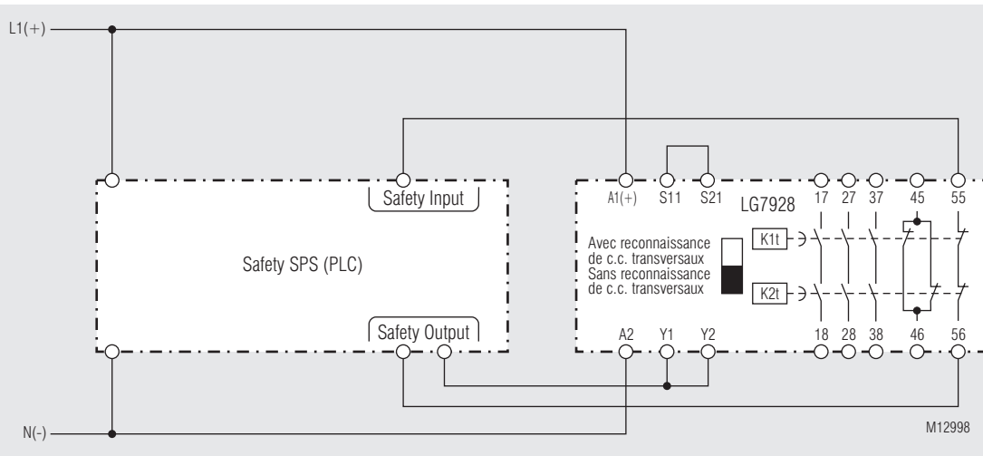
AP de sécurité avec LG 7928, sans reconnaissance de cc transversaux, convient jusqu'à SIL 2, Performance Level d, Cat. 3
