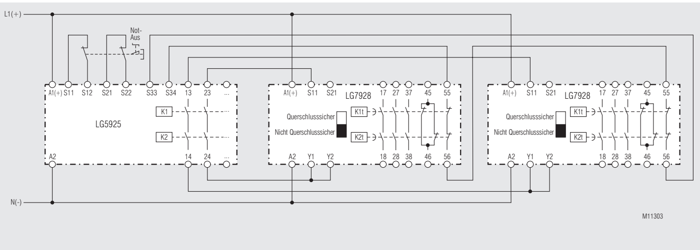
LG 5925 mit zwei LG 7928, nicht querschlosssicher, geeignet bis SIL 2, Performance Level d, Kat. 3
