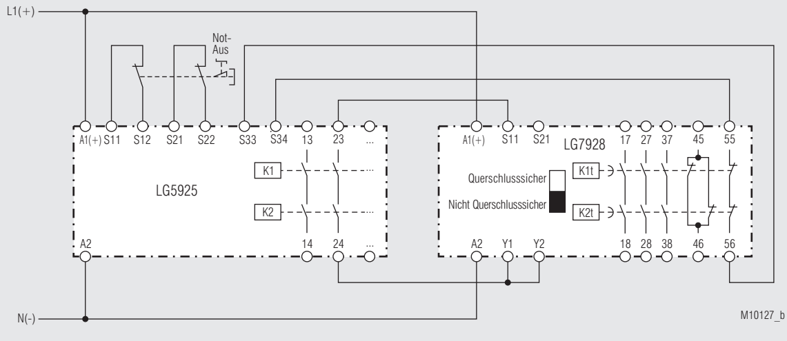
LG 5925 mit LG 7928, nicht querschlosssicher, geeignet bis SIL 2, Performance Level d, Kat. 3
