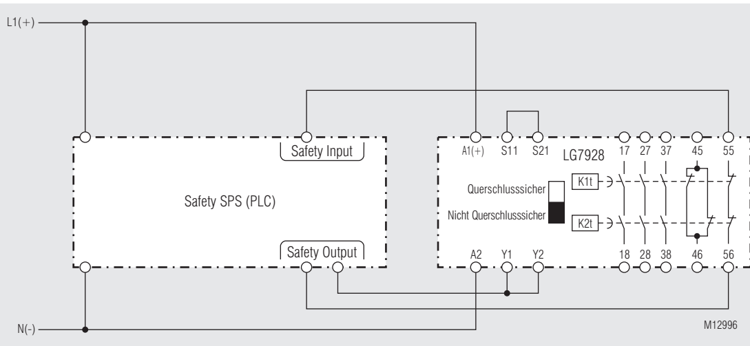
Safety SPS mit LG 7928, nicht querschlosssicher, geeignet bis SIL 2, Performance Level d, Kat. 3
