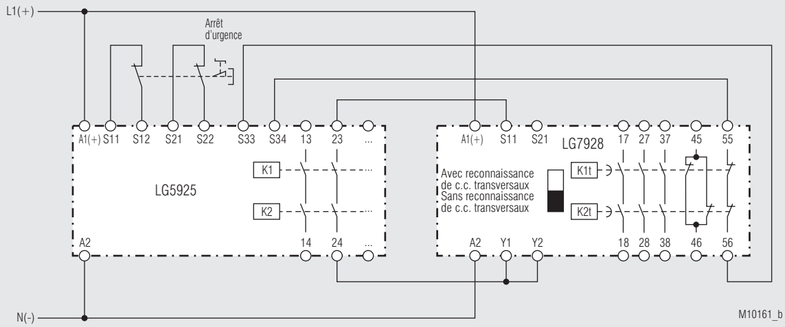
LG 5925 avec LG 7928, sans reconnaissance de cc transversaux, convient jusqu'à SIL 2, Performance Level d, Cat. 3
