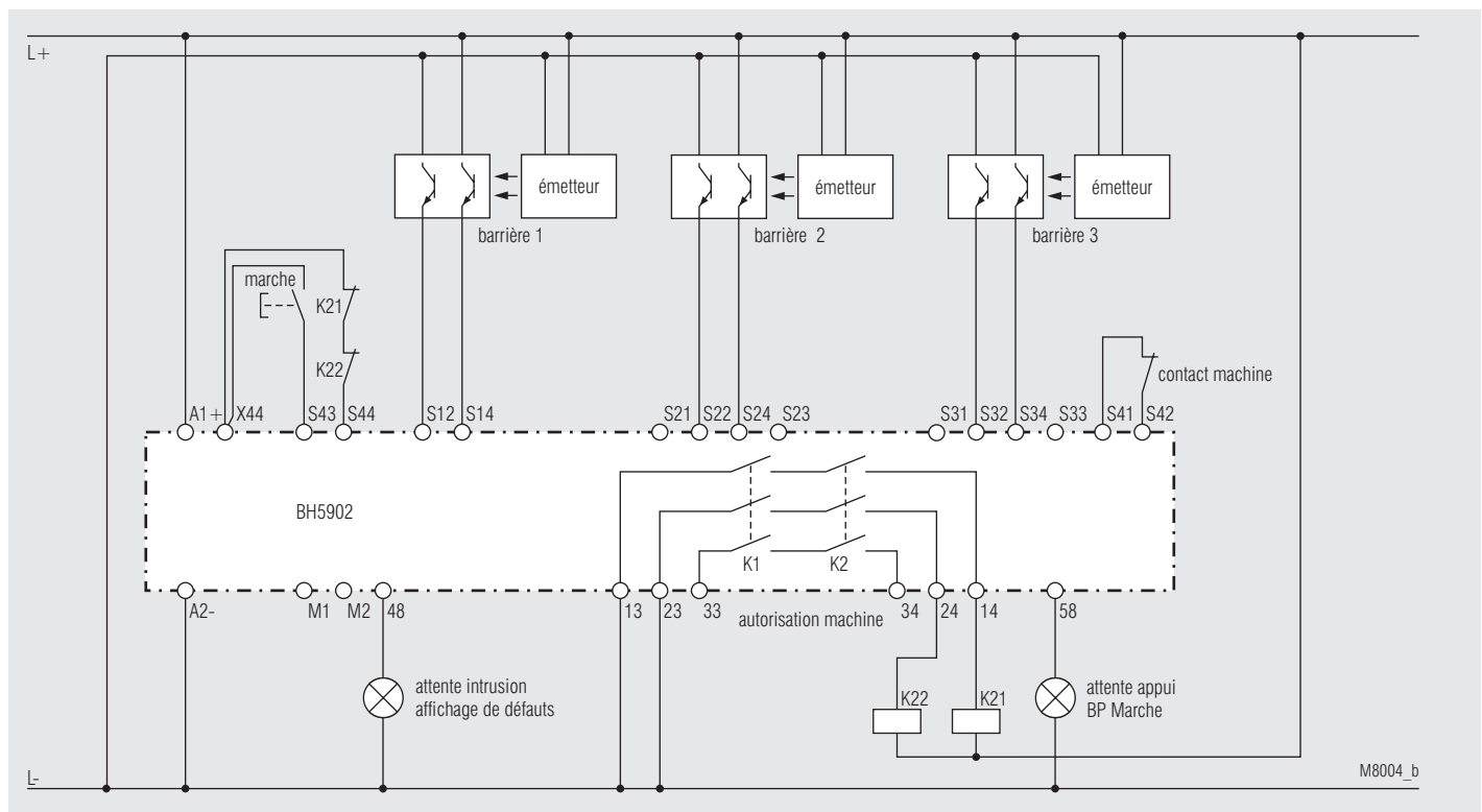
Schéma 7: Fonctionnement d'intrusion avec 3 barrières et relayage par contacteurs, 2 canaux (Schéma avec renfort de contacts pouvant être utilisé pour le Muting)
