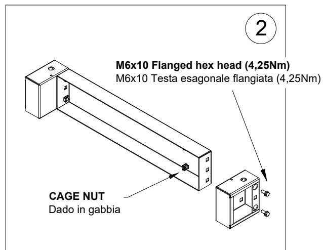
CAGE NUT M6 Dado in gabbia M6
