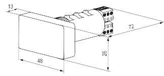
Fig. 3 Dimensions
