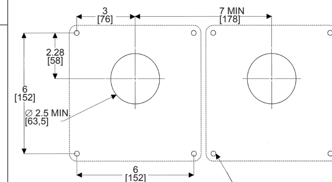
Fig. 6 CUT-OUT PANEL OPENING/DÉCOUPE DE PANNEAU/ CORTE EN EL PANEL 60 A/100 Angle Adapter/Adaptateur coudé 60/100 A Adaptador en ángulo 60/100 A
