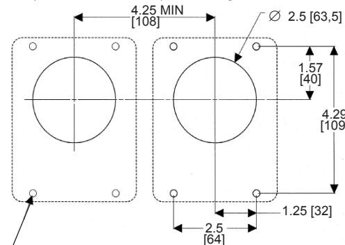
CUT-OUT PANEL OPENING/DÉCOUPE DE PANNEAU/CORTE EN EL PANEL 30 A Angle Adapter/Adaptateur coudé 30 A/Adaptador en ángulo 30 A
