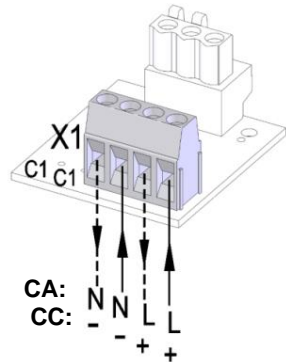
Raccordement de la tension de service
