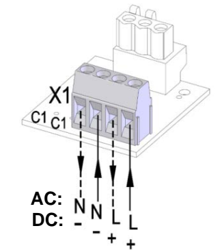
Betriebsspannungsanschluss
