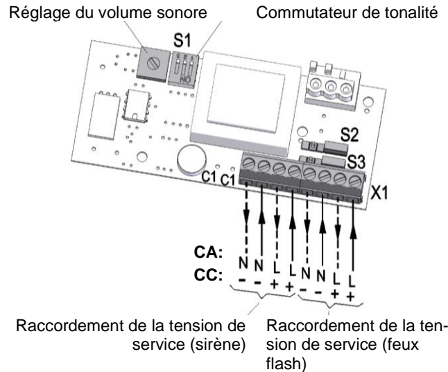
Commutateur de tonalité Raccordement de la tension de service (sirène) Raccordement de la tension de service (feux flash)
