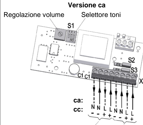
Collegamento tensione operativa dal segnalatore acustico Collegamento tensione operativa della luce flash
