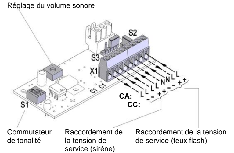
Raccordement de la tension de service (sirène) Raccordement de la tension de service (feux flash)
