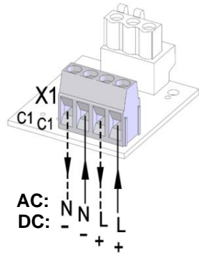
Collegamento tensione operativa
