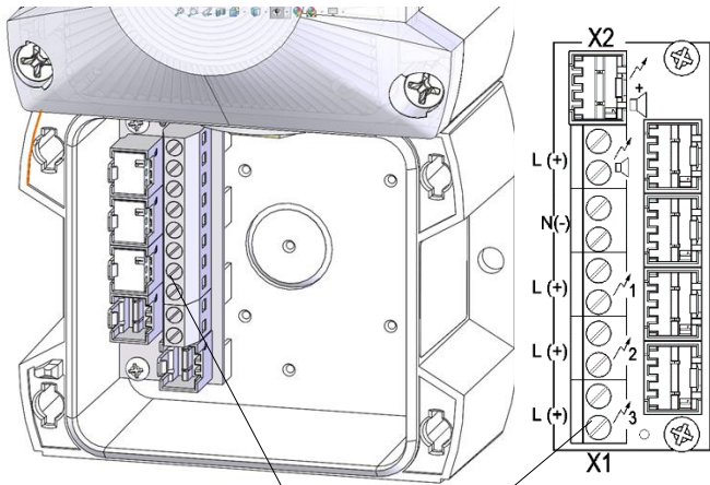
Соединительный зажим (X1)
