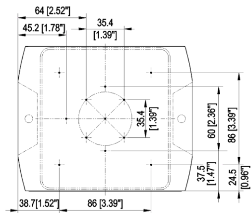
Схема расположения отверстий внутри корпуса
