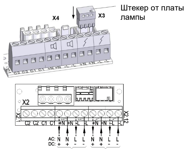
Подключение рабочего напряжения излучателя звука Подключение рабочего напряжения лампы
