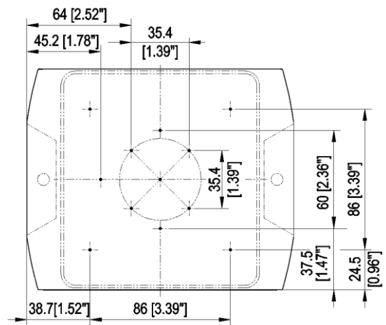
Schema forature interne all'alloggiamento
