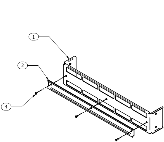
STEP 1 - DIN rail assembly
