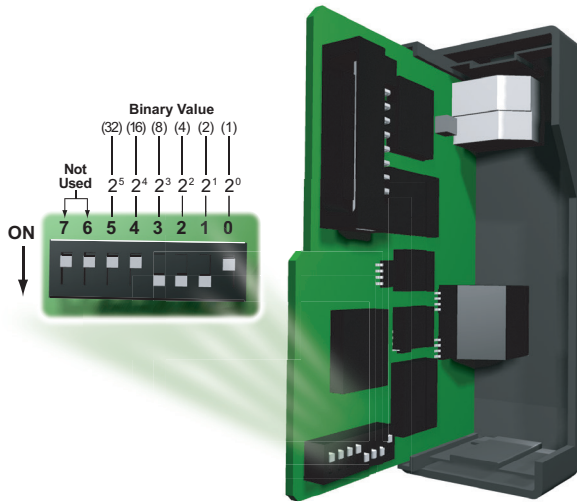
H2-ERM(100)/H2-EBC Module
