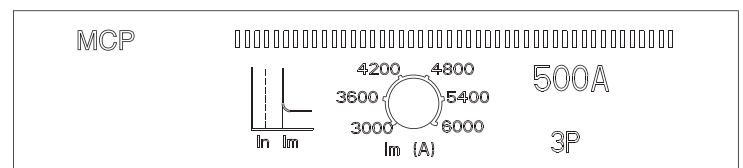
<Fig. 8> Type of trip units / Tipo de unidad de disparo / Type de déclencheurs
