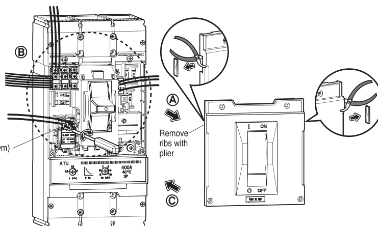
<Fig. 6> Accessory installation / Instalación de accesorio / Installation des accessoires
