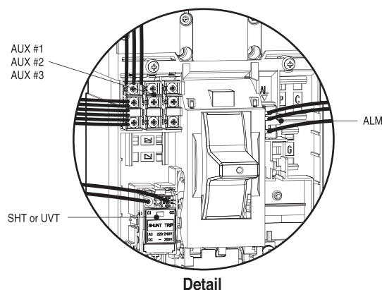
<Fig. 7> Control Wiring Installation / Instalación de cable de control / Installation de câblage de contrôle
