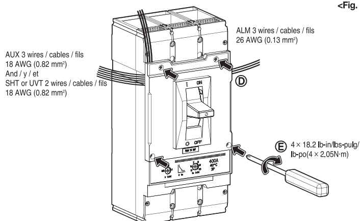
<Fig. 7> Control Wiring Installation / Instalación de cable de control / Installation de câblage de contrôle
