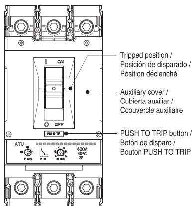
<Fig. 4> Circuit Breaker Manual Controls / Control manual del interruptor / Commande manuelle du Disjoncteur
