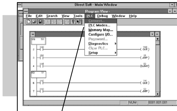
Menu Options
