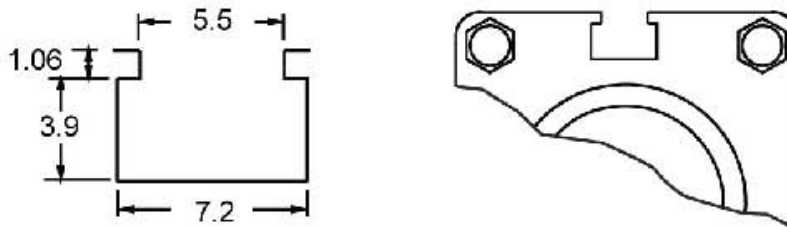
GROOVE DIMENSIONS
