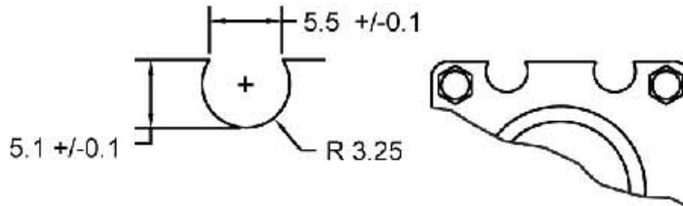
GROOVE DIMENSIONS
