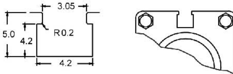
GROOVE DIMENSIONS
