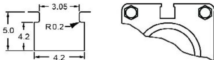
GROOVE DIMENSIONS
