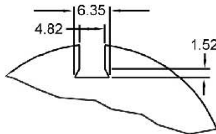
GROOVE DIMENSIONS
