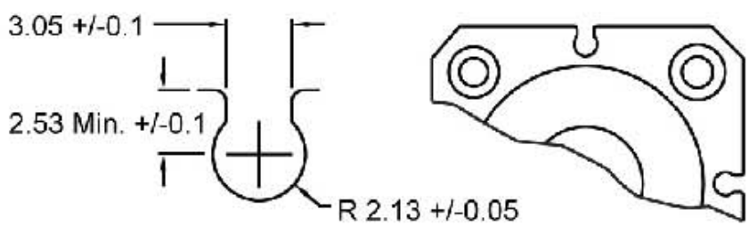
GROOVE DIMENSIONS
