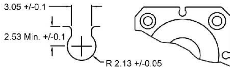
GROOVE DIMENSIONS
