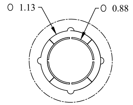
DETAIL Y TYP (10)
