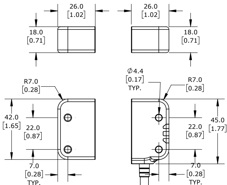
ACTUATOR
