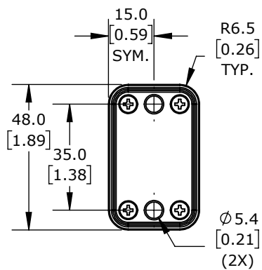
ACTUATOR
