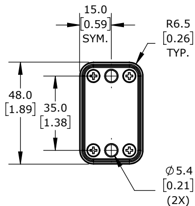
ACTUATOR
