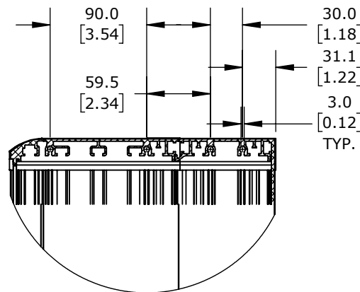
SECTION B SCALE 1 : 5
