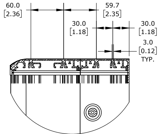
SECTION B SCALE 1 : 4
