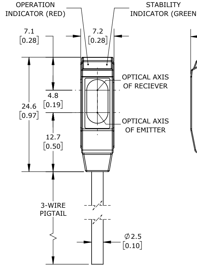
SENDER RECIEVER
