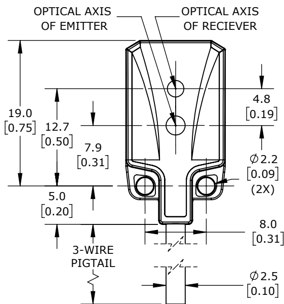
SENDER RECIEVER
