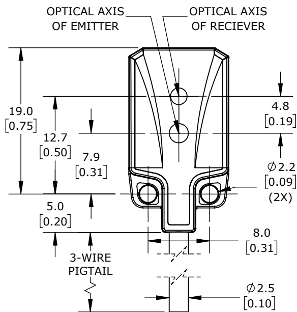
SENDER RECIEVER
