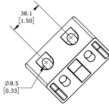
VIEW A-A
